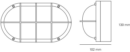
8122 H: 130 mm x W: 230 mm
