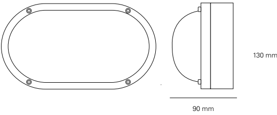
8120 H: 130 mm x W: 230 mm
