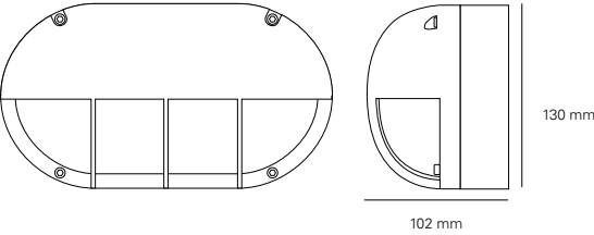
8125 H: 130 mm x W: 230 mm
